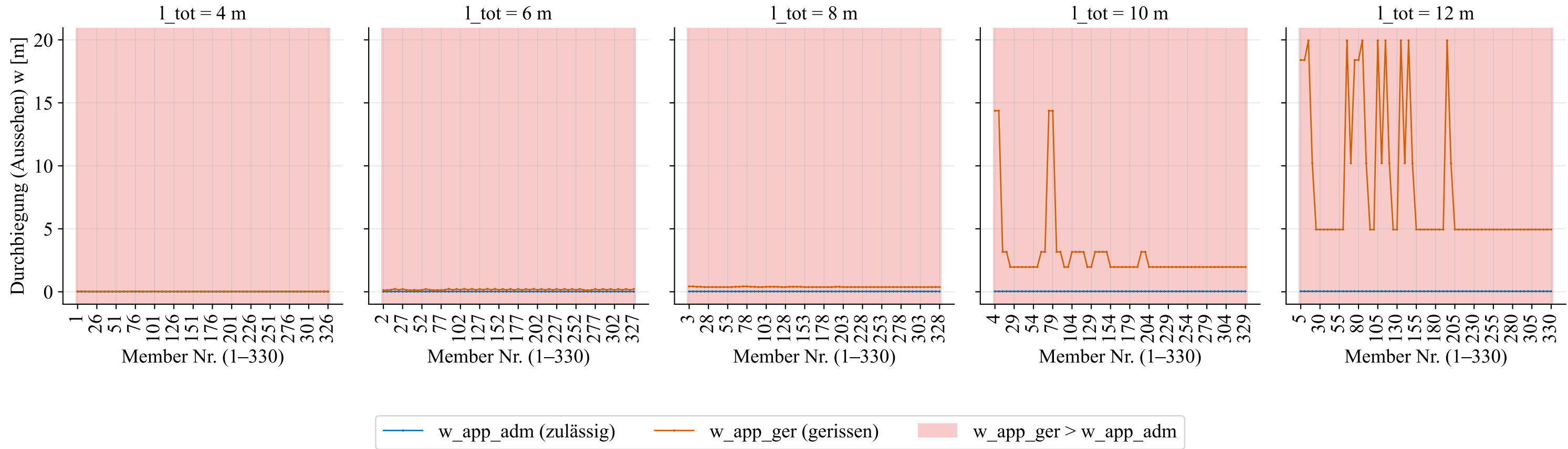
Durchbiegung w_{app\_adm} (zulässig) vs. w_{app\_ger} (gerissen) je Member, kategorisiert nach Spannweite (Members_rc_rib_simple_V3)
